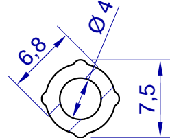
Snitt M8-M8
