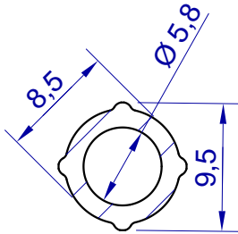
Snitt M10-M10
